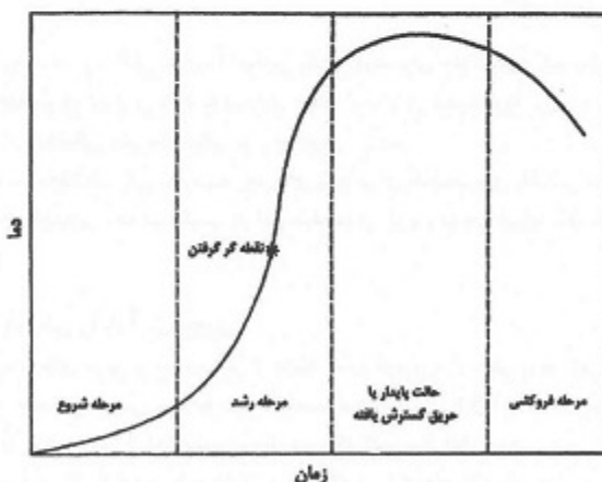
شکل پ-۲-۲: منحنی استاندارد رشد آتش‌سوزی
